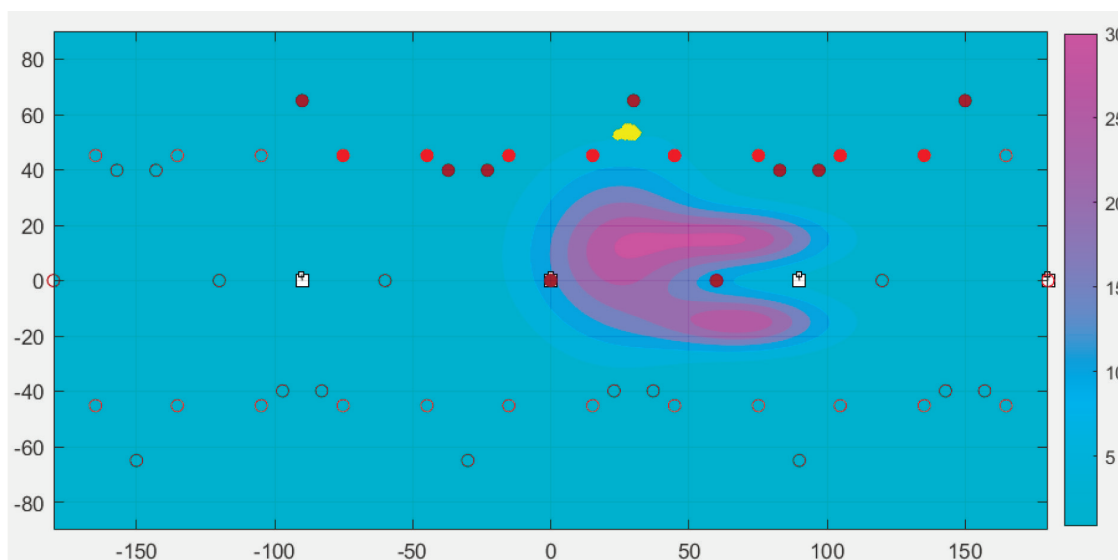
Развертка компьютерной имитационной модели низкоорбитального контроля ионосферы
