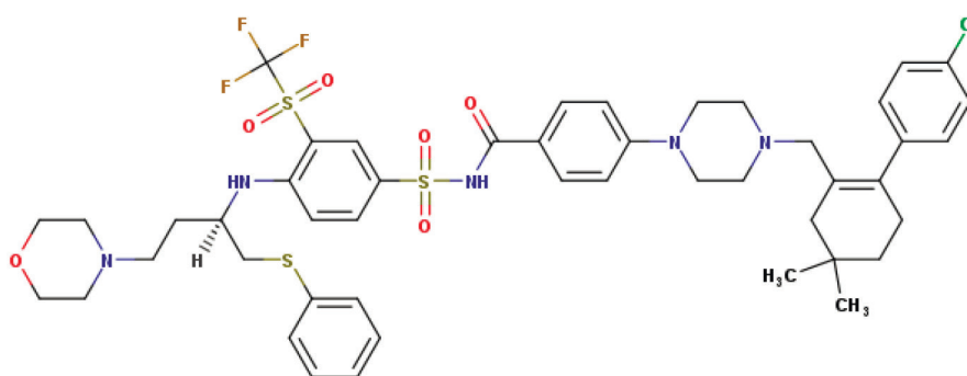
Химическая структура препарата «Навитоклакс»
