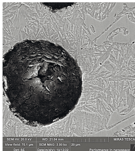
Структура разработанного чугуна CADi (×3000)
