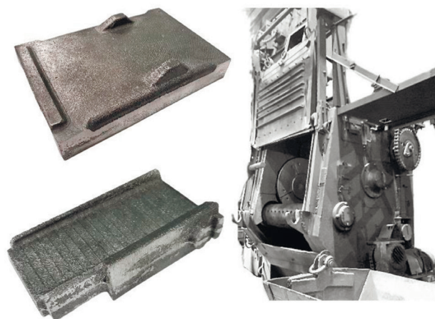
Изделия, полученные из чугунов CADi
