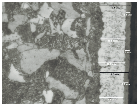
Белый и оксидный слои на штоке из стали 40Х, полученные методом оксинитрирования
