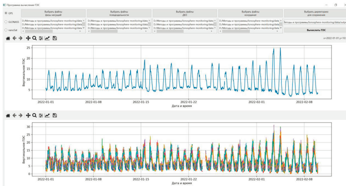
Вычисление полного электронного содержания ионосферы
